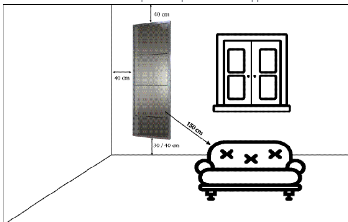
Installation préconisée dans le cadre d'une utilisation optimale de votre appareil.
